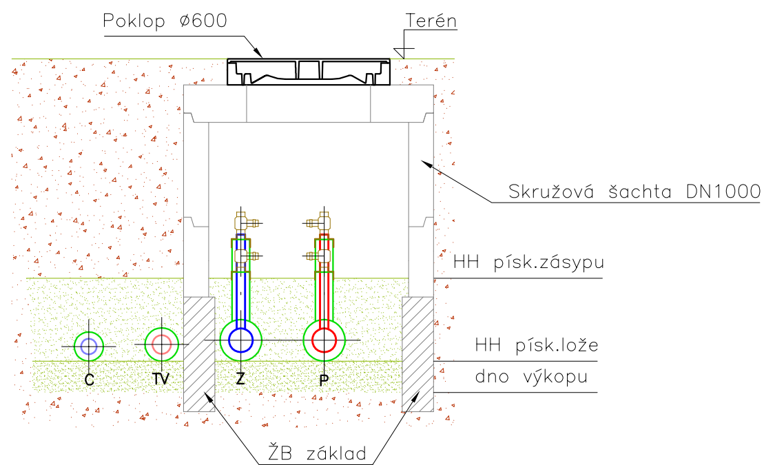
ŘEZ A-A
