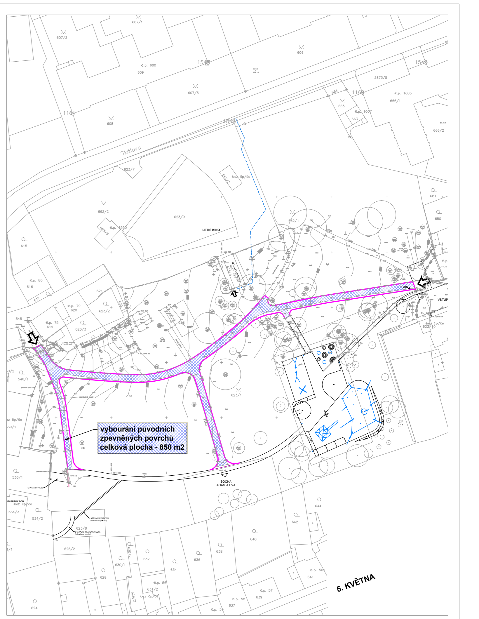
BOURÁNÍ - SITUACE 1:1000
